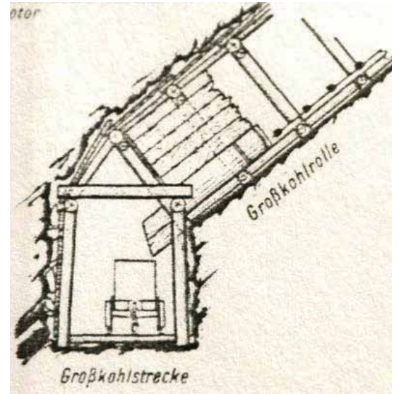
Stollenausbau mit Holzstempeln auf den entsprechenden Sohlen, Weithofer 1920
